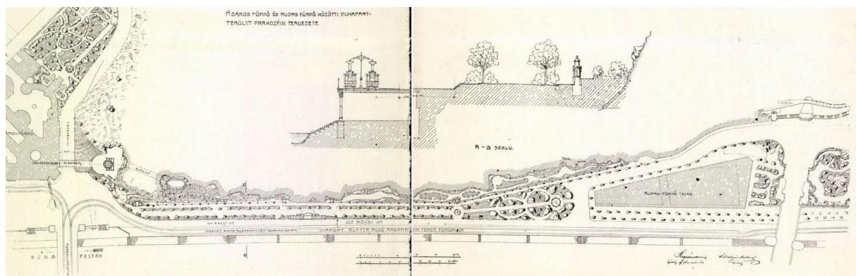
7. ábra A Gellért hegy lábánál húzódó sétány terve (Forrás: Építő Ipar 1907, 31. évf. 362-363, képek összekapcsolása: a szerző, 2022)
