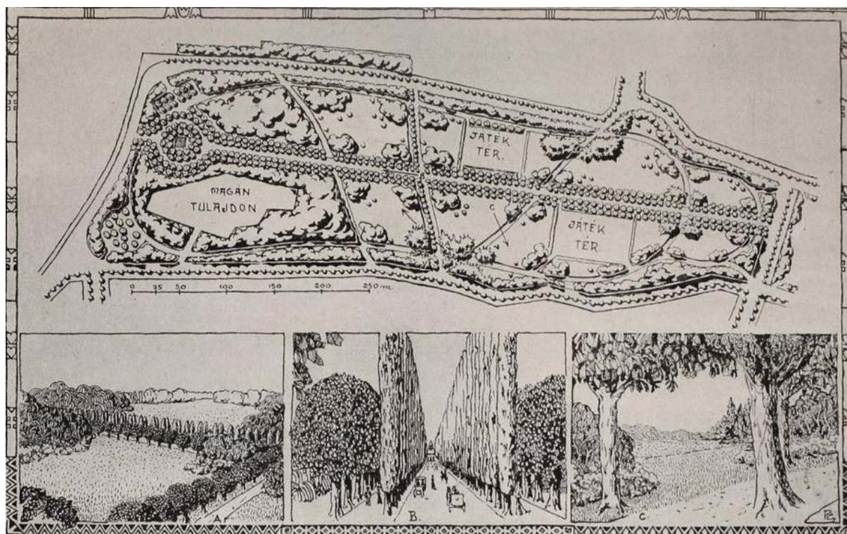
34. ábra Ifj. Pecz Ármin terve a győri Rábca-part parkjának 8. kertjéhez, 1910 (kép forrása: Kertészeti Lapok 1911,78)
