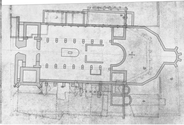
9. ábra: A bazilika alaprajza a prépostságéra ráhelyezve, saját szerkesztés
