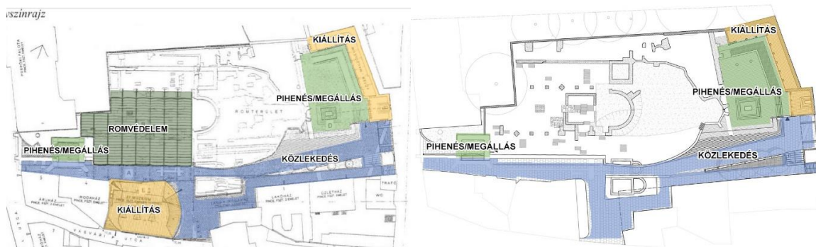
23. ábra: A tervezői elképzelés funkciószámja; Saját szerkesztés; forrás: Oltai, 2000
