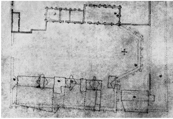
8. ábra: 1712-es prépostsági alaprajz forrás: INT-05
