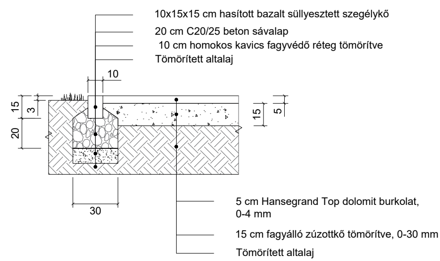
S1 10 CM HASÍTOTT BAZALT SÜLLYESZTETT SZEGÉLYKŐ gyep - stabilizált burkolat esetén
