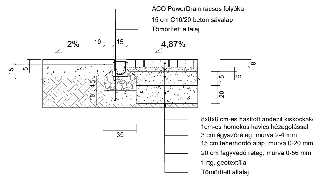
stabilizált burkolat - gépjármű és gyalogos forgalom számára kiskockakő burkolat esetén
