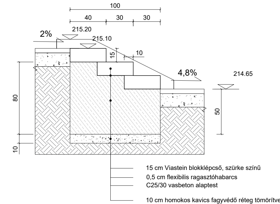
LÉPCSŐ METSZET (főtengelyben található lépcső) M=1:25
