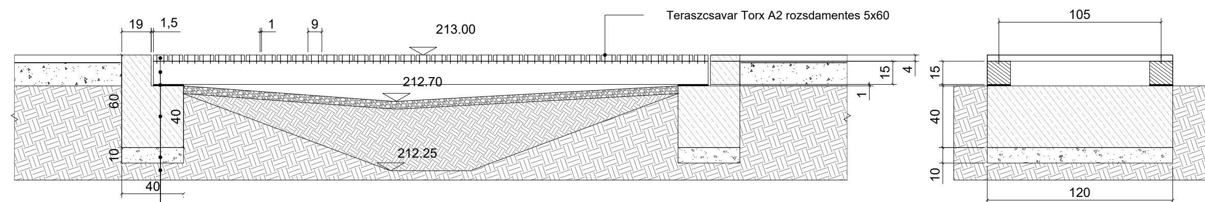
FA HÍD METSZET M=1:50
