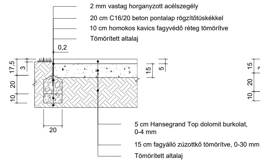
S2 FÉMSZEGÉLY gyep - stabilizált burkolat esetén
