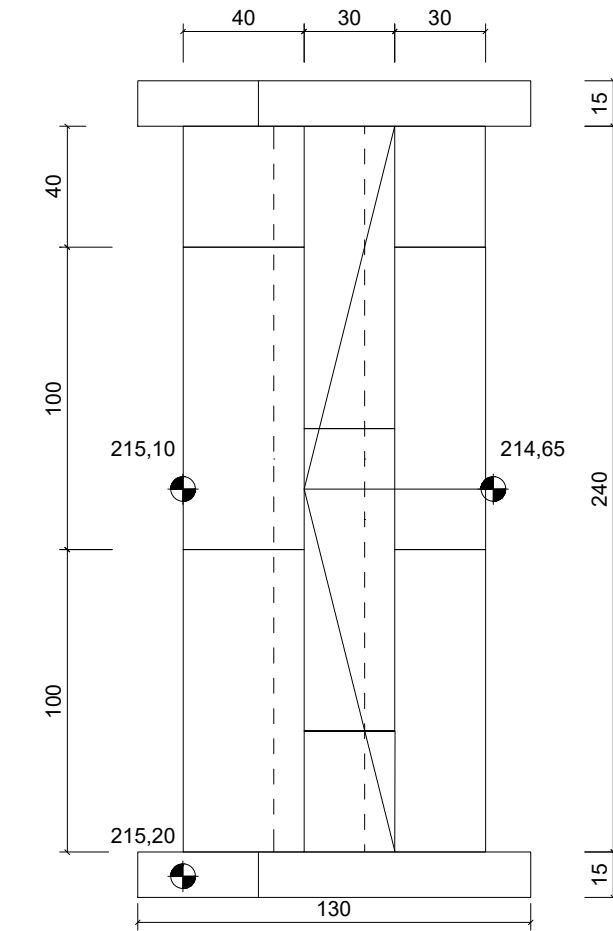
LÉPCSŐ FELÜLNÉZETE (főtengelyben található lépcső) M=1:25
