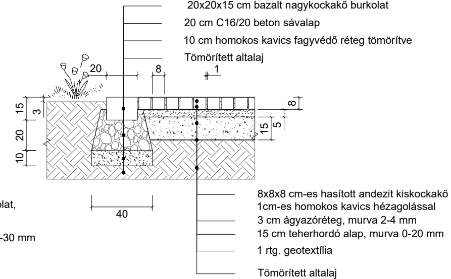
S3 SÜLLYESZTETT NAGYKOCKAKŐ SZEGÉLY növényágyás - gyalogos forgalom számára kiskockakő burkolat esetén
