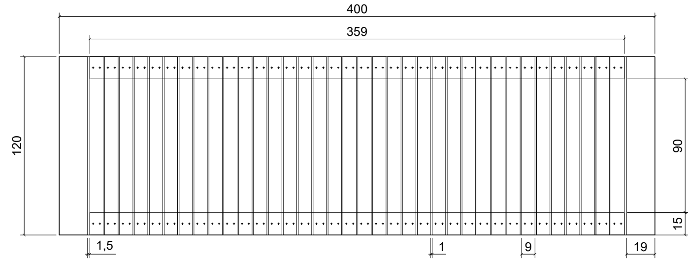
FA HÍD METSZET M=1:50
