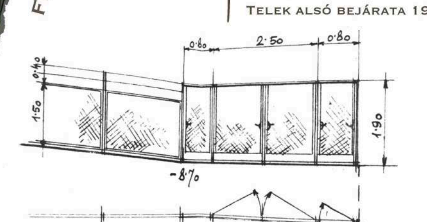
Fillér utcai kerítés és bejárat 1:100
