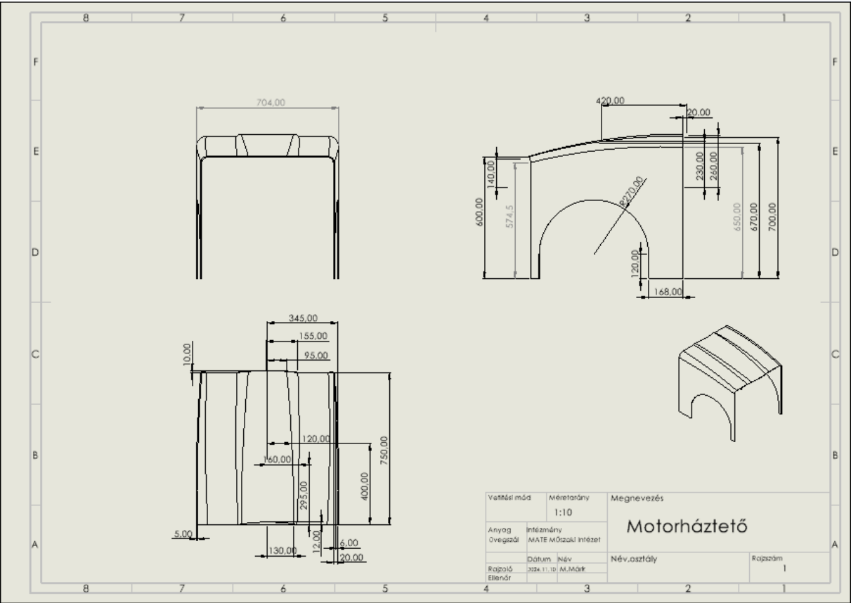
2.Melléklet: Motorháztető műhelyrajza (Forrás: saját munka)
