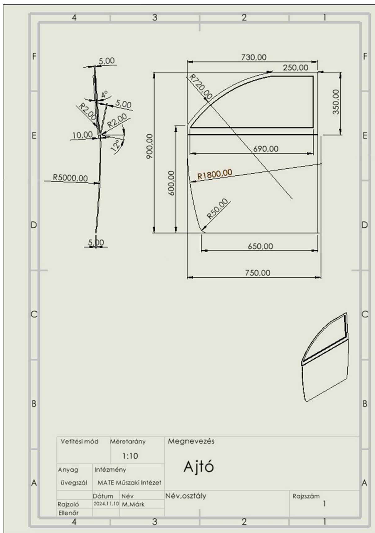
1.Melléklet: Ajtó műhelyrajza (Forrás: saját munka)
