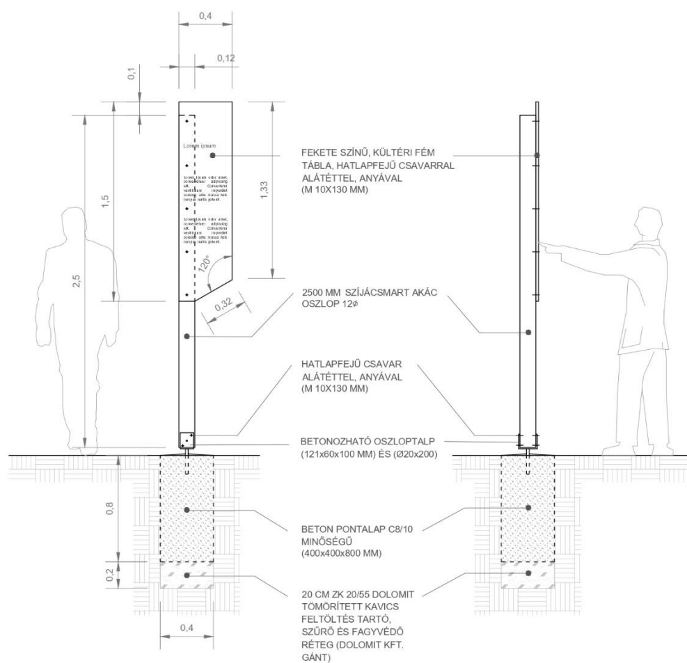
11. ábra Tervezett objektum (1:20) Forrás: saját ábra
