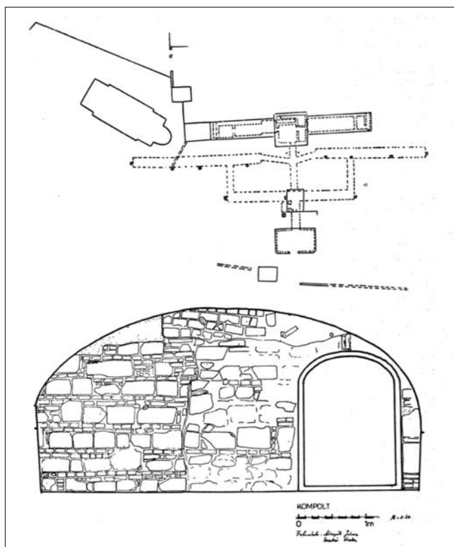
7. melléklet: Az uradalmi pince alaprajza és bejáratának rajza (BAKÓ 1994, 181.)
