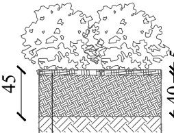
Zöldfelület cserjesáv alatt M=1:50
