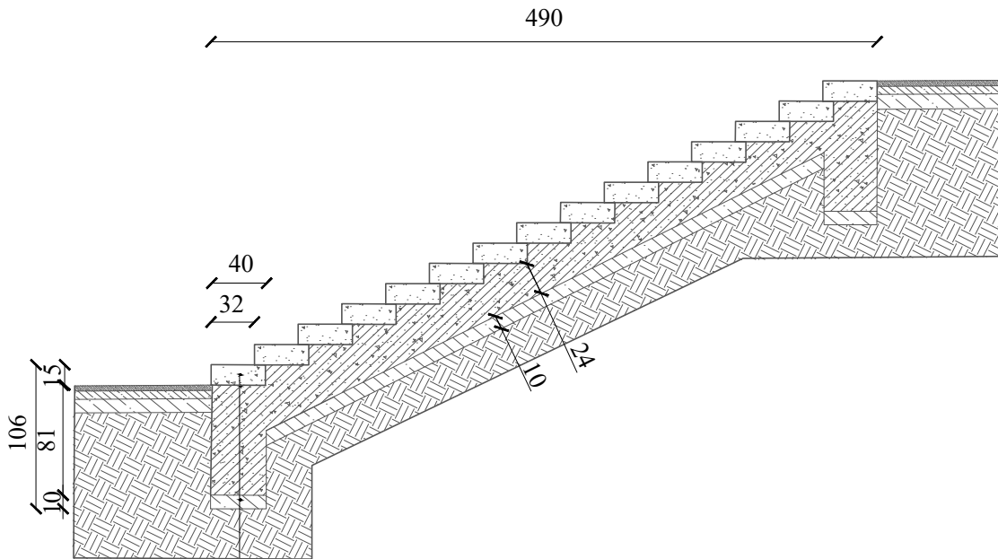
Lépcső metszet M=1:50
