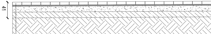
Térkő burkolat - Via Casa Antik egyedi láva-antracit színben autós burkolat M=1:50
