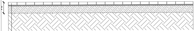
Térkő burkolat - Via Casa Antik egyedi láva-antracit színben gyalogos burkolat M=1:50
