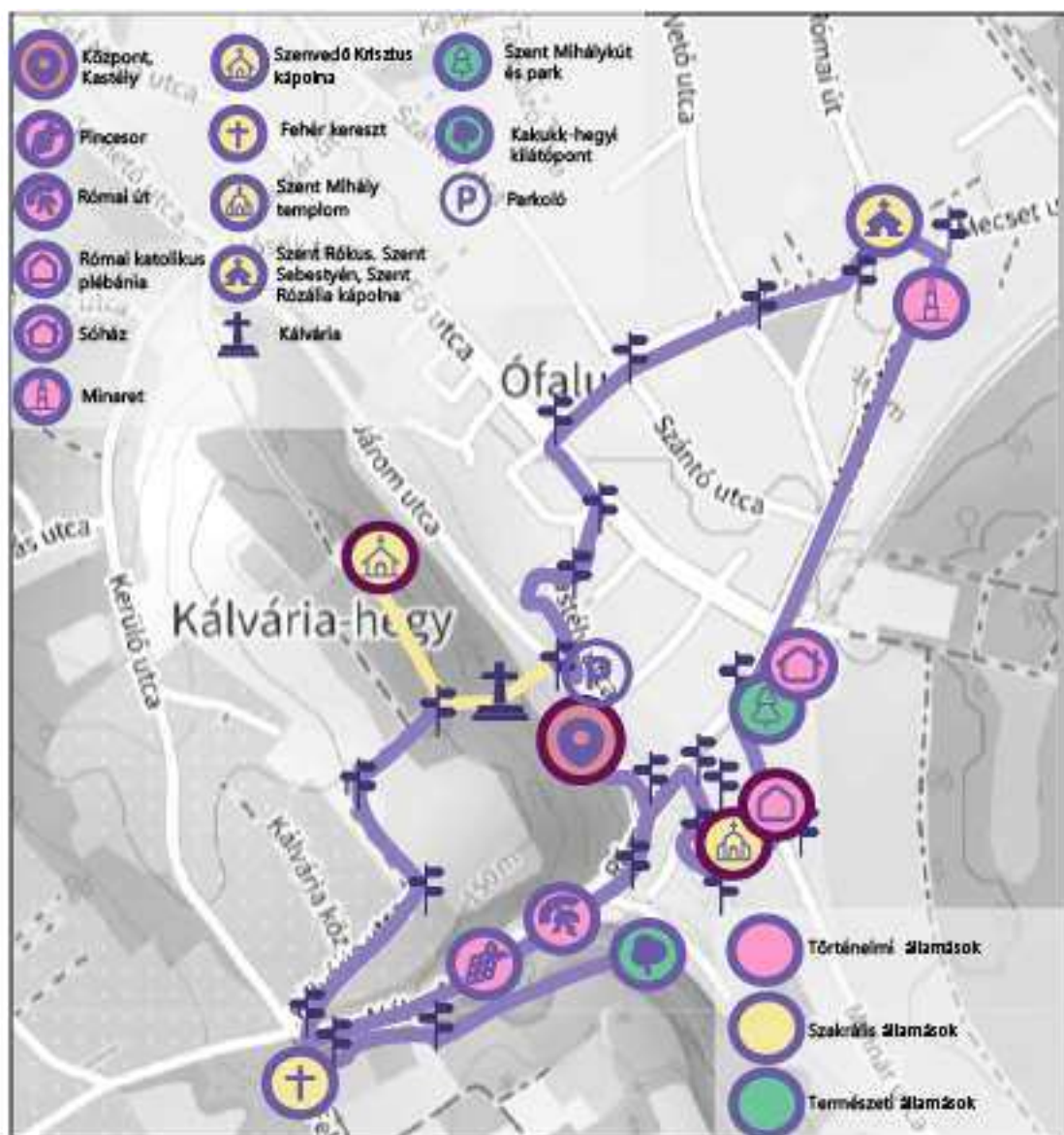
52. ábra Turisztikai útvonal terve
